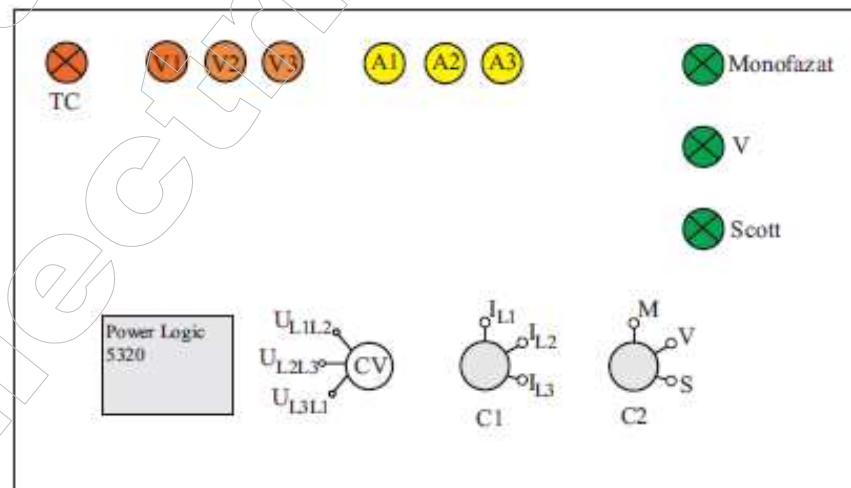
Figura 10. Panou substații de tracțiune.
