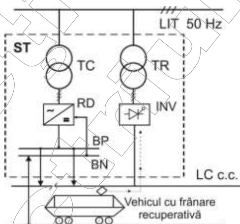
Figura 3. Substație de tracțiune pentru recuperare de energie.
