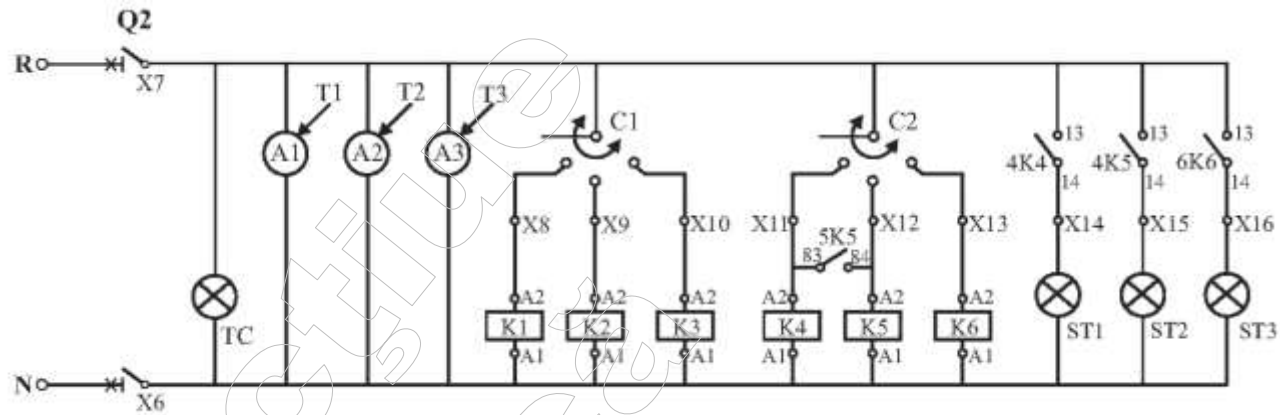
Figura 9. Schema de comandă.
