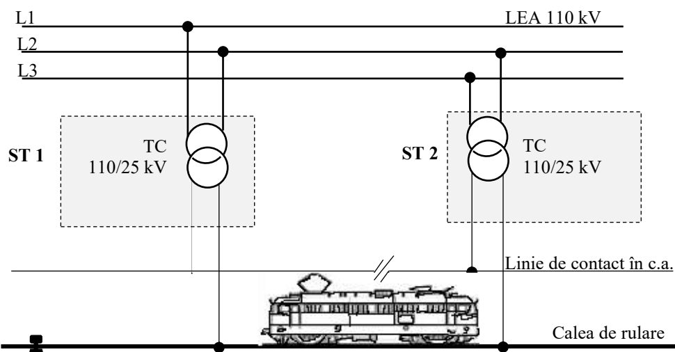
Figura 4. Sistem de tracțiune în c.a. monofazat de 50 Hz.
