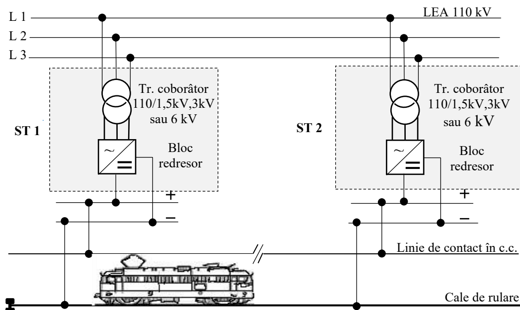
Figura 2. Sistemul de tracțiune în c.c.
