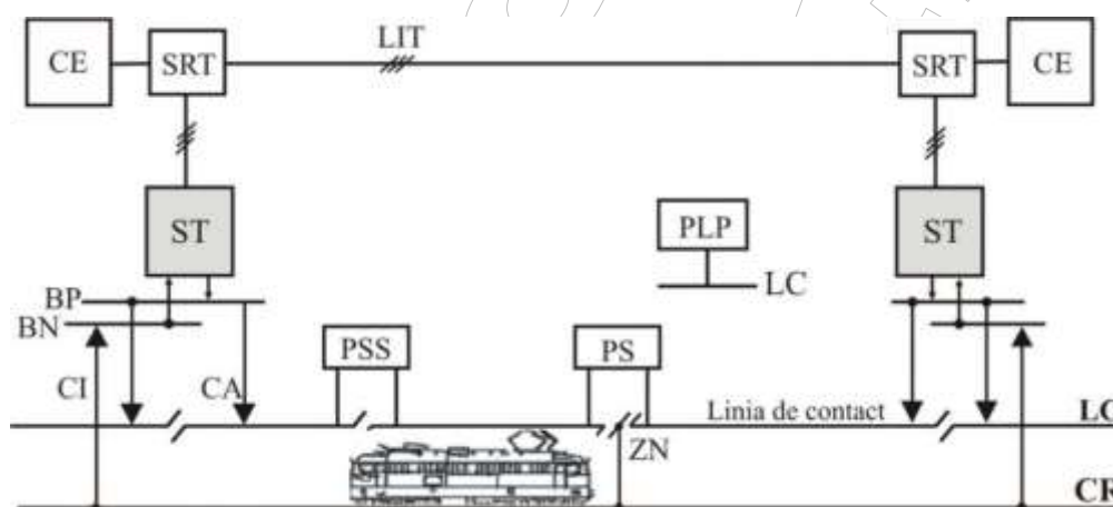
Figura 1. Schema generală a unui sistem de tracțiune electrică.
