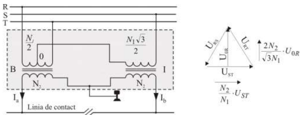
Figura 6. Substație cu transformatoare în montaj Scott.
