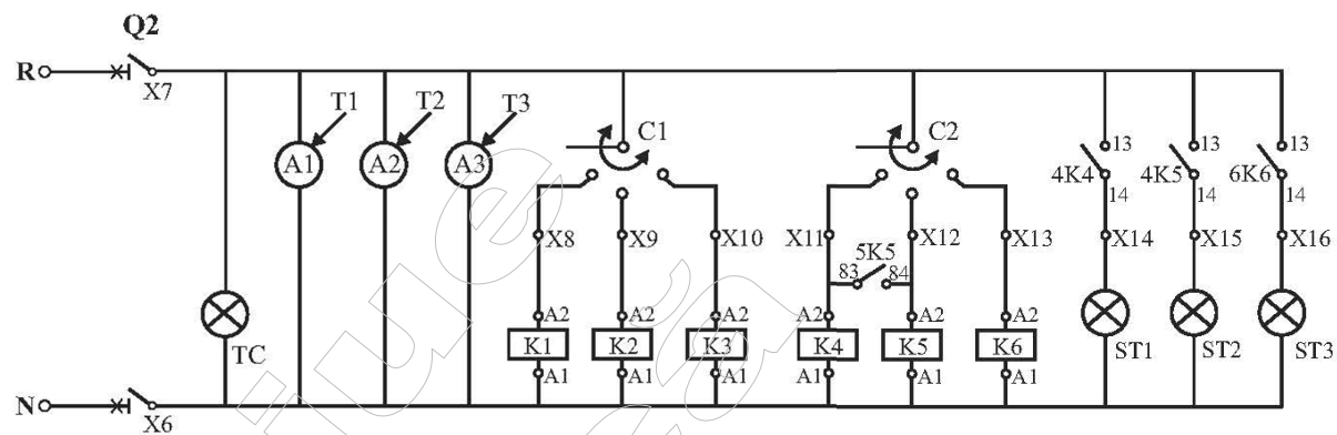
Fig. 9. Schema de comandă.
