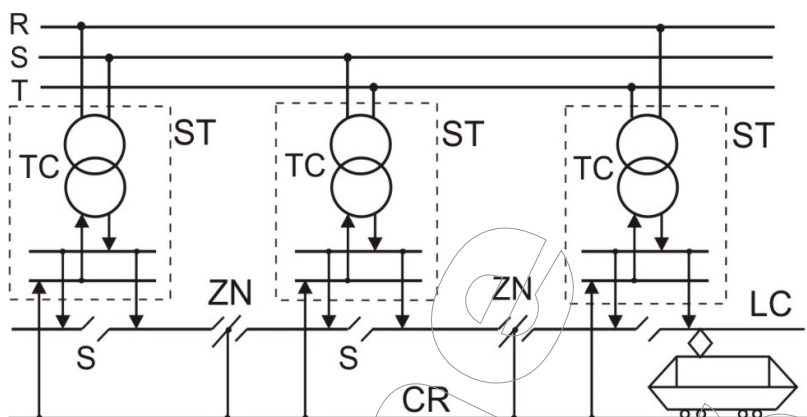
Fig. 5. Legarea ciclică a substațiilor.
