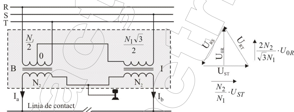
Fig. 6 Substație cu transformatoare în montaj Scott.
