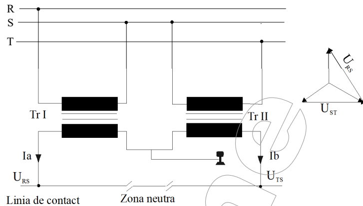
Fig. 7. Substație cu transformatoare în montaj în V.
