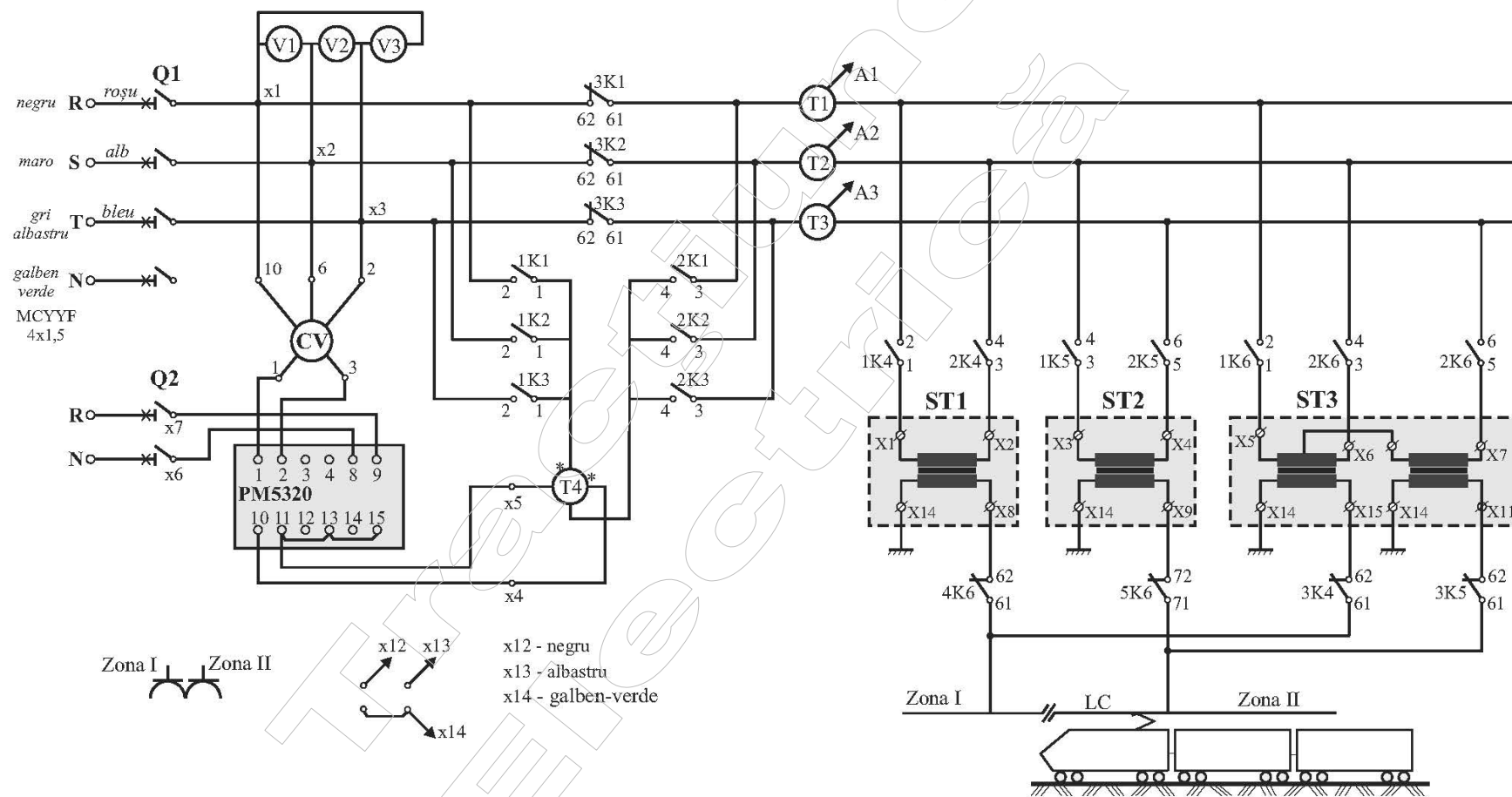
Fig. 8. Schema de forță a standului de laborator.
