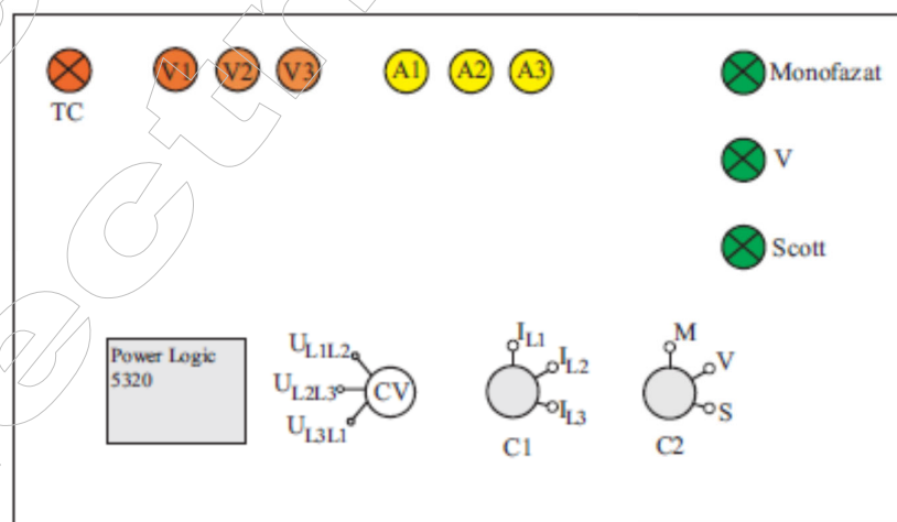
Fig. 10. Panou substații de tracțiune.
