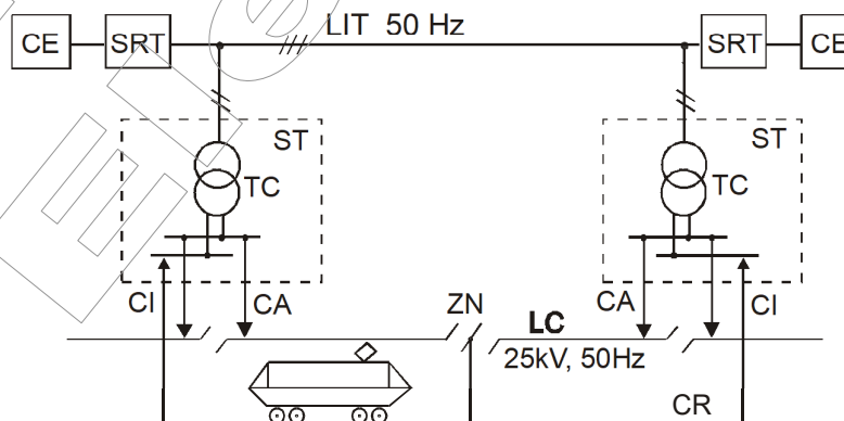
Fig. 4. Sistem de tracțiune în c.a. monofazat de 50 Hz.
