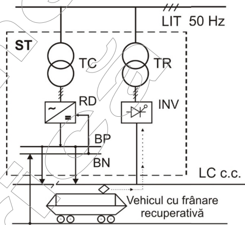
Fig. 3 Substație de tracțiune pentru recuperare de energie.
