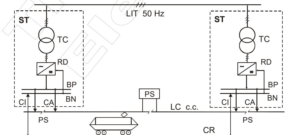
Fig. 2. Sistemul de tracțiune în c.c.
